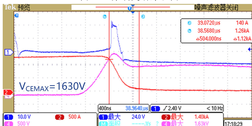
图 14a 不带分级关断
