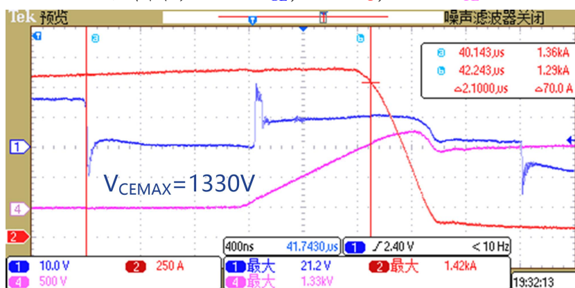
图 14b 带分级关断
