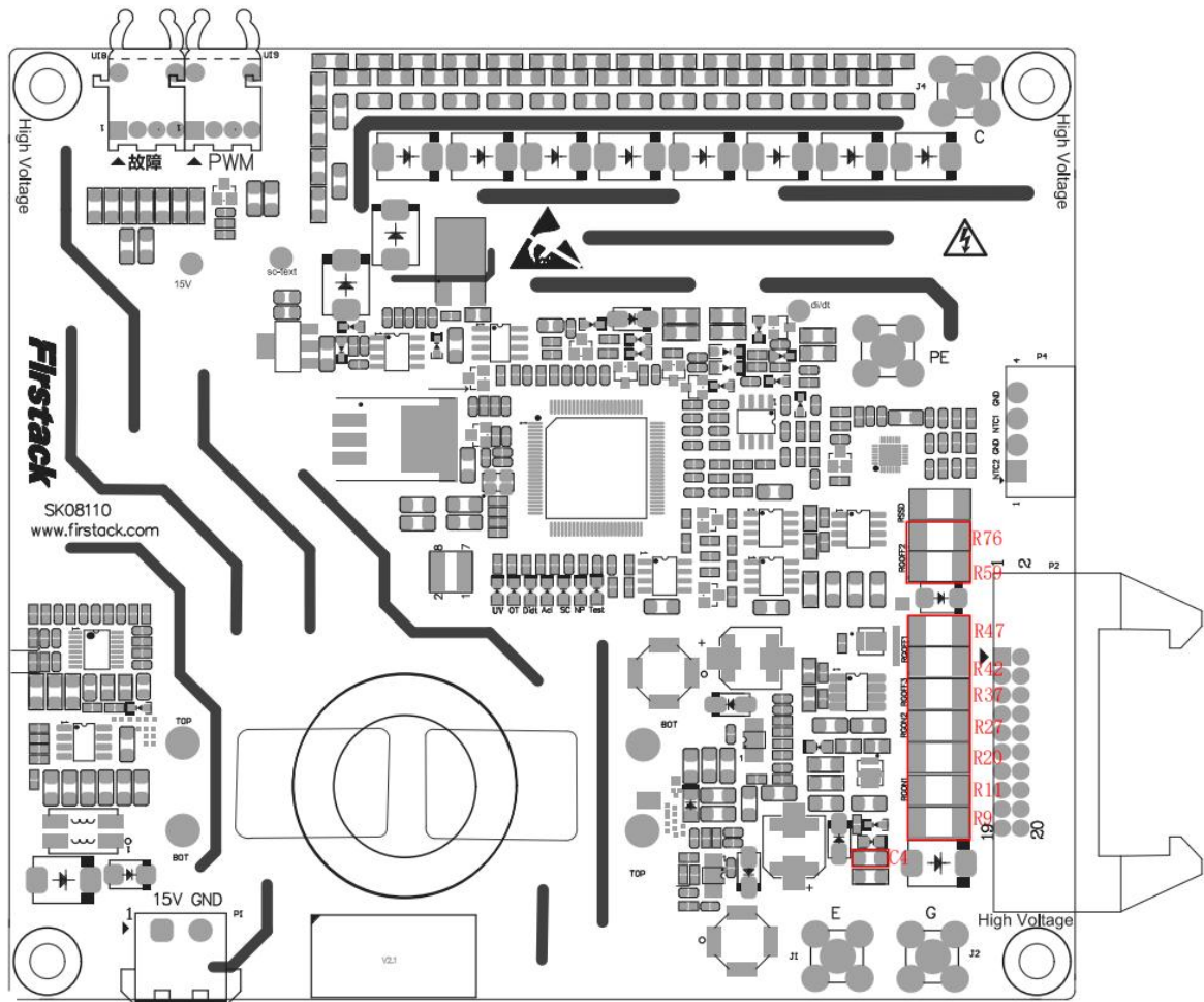
图 19 门极电阻位置指示图
