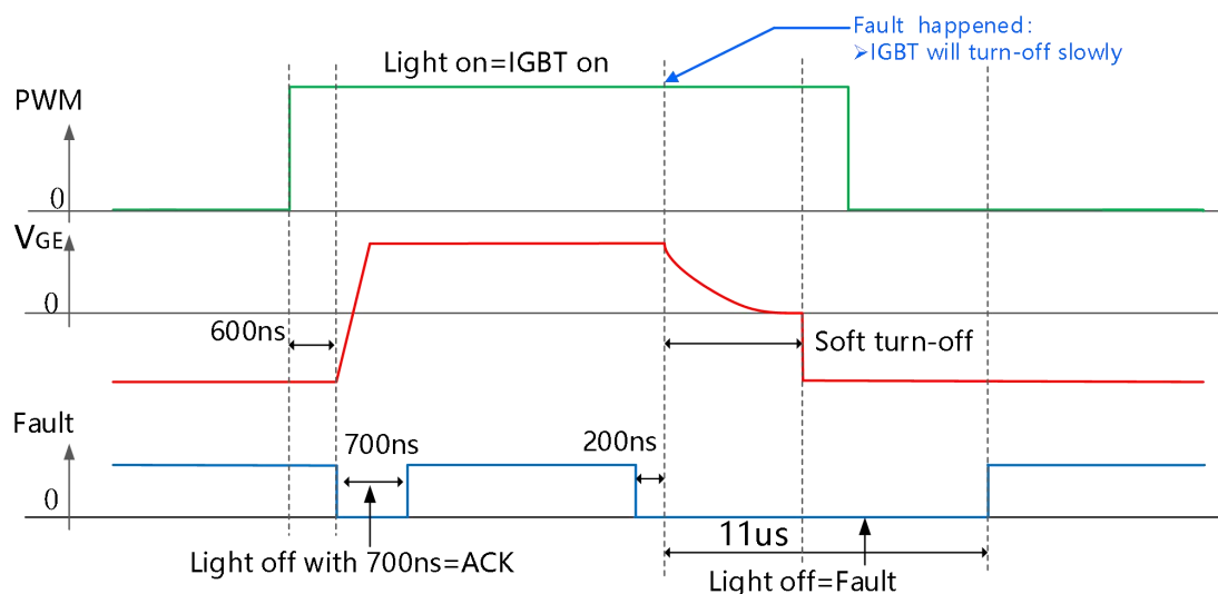
图 16b 故障情况下图
