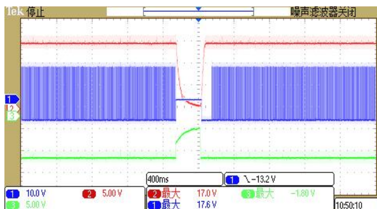
图 15 GE 短路
