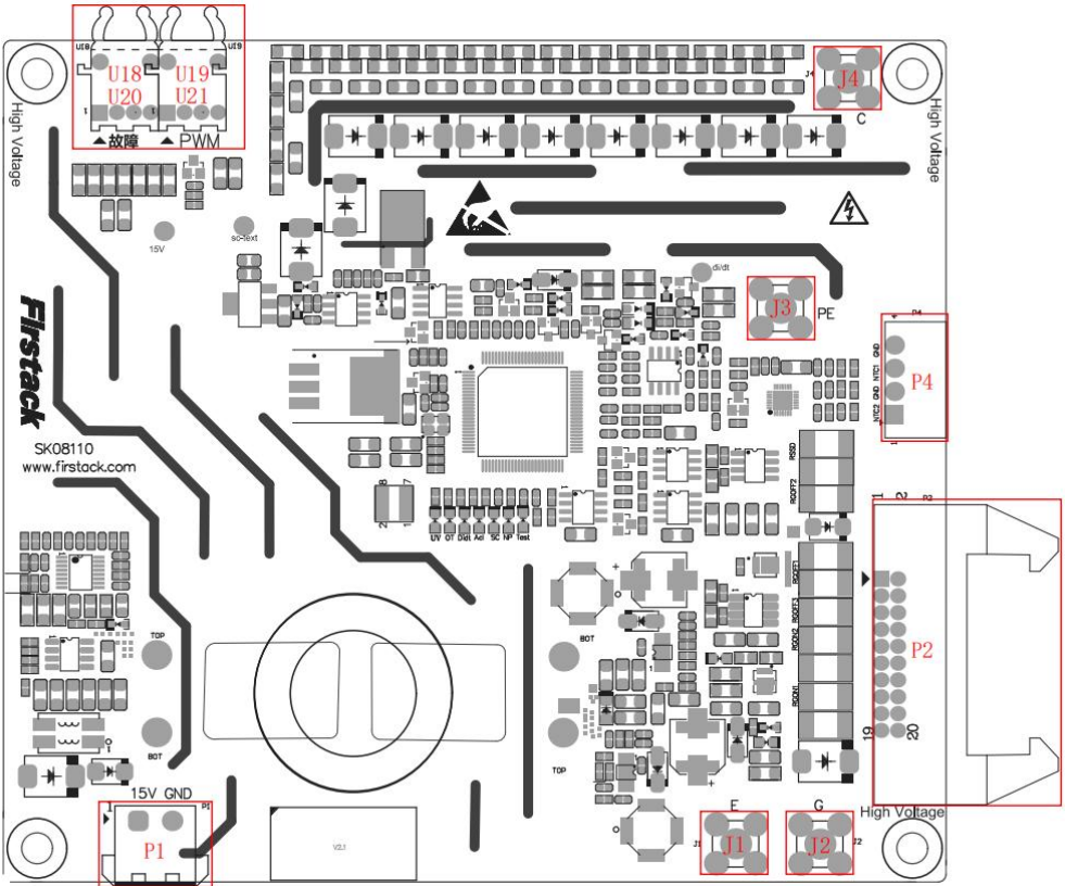
图 5 SK08110 驱动器接口图
