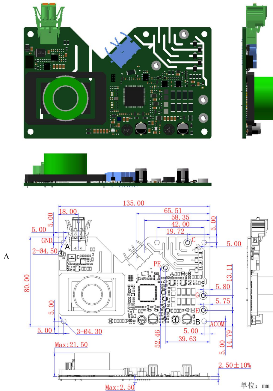
图 3 1FSS0560 尺寸图
