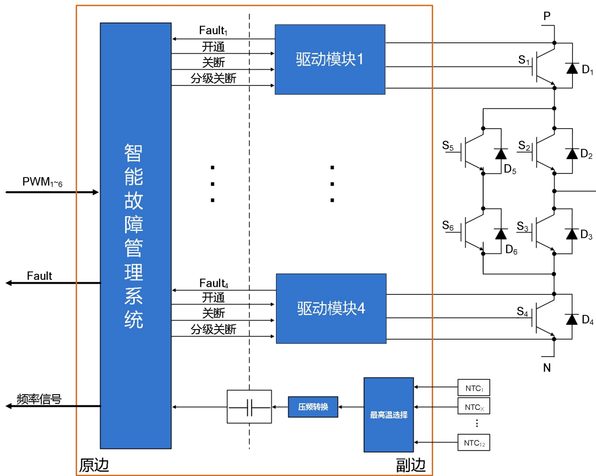
图2 功能框架图
