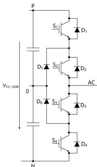
图 11 ANPC I 型三电平拓扑
