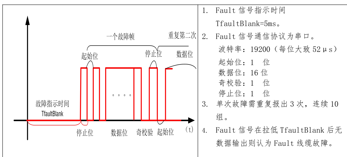
图 10 故障通信时序图
