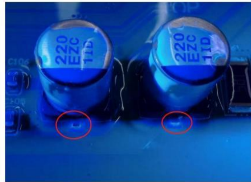
贴片电容引脚喷涂，表面可不喷
