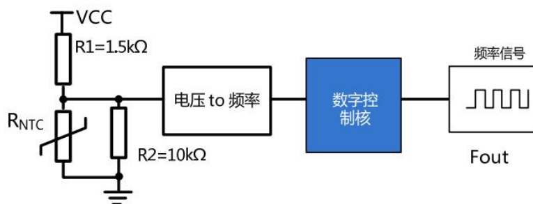
图 7 温度监测原理图
