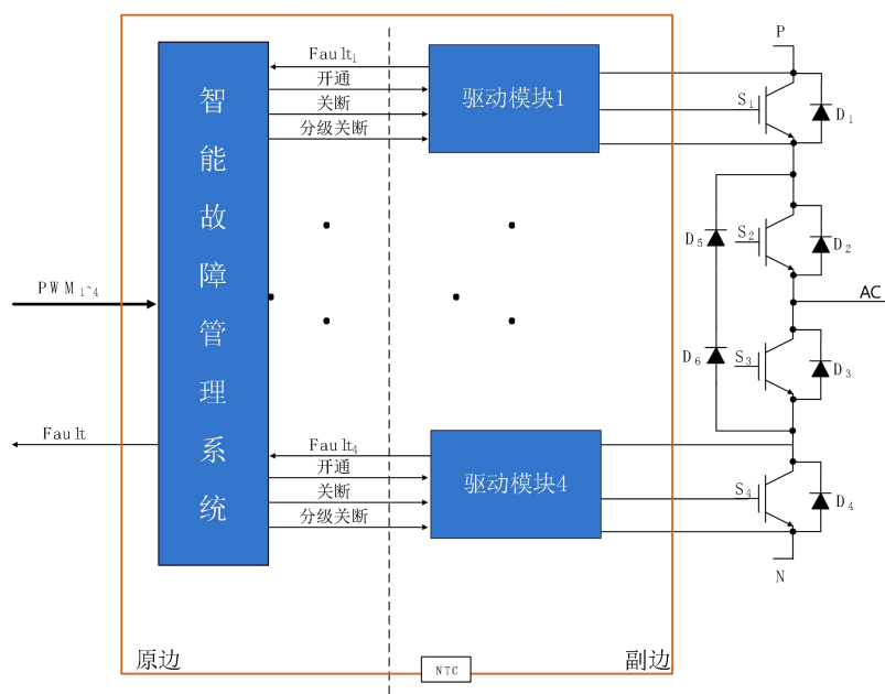
图 12 智能故障管理系统
