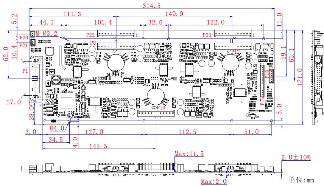
图 3 尺寸图
