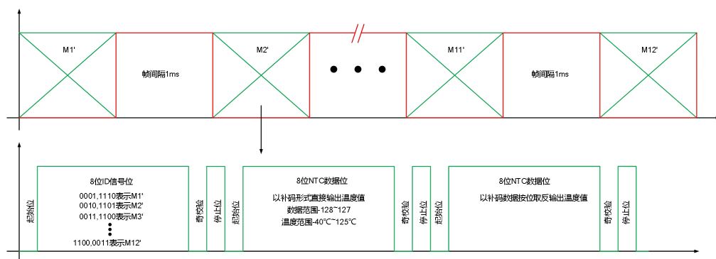
图 8 温度监测原理图
