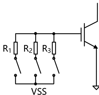
图 6 分级关断原理图
