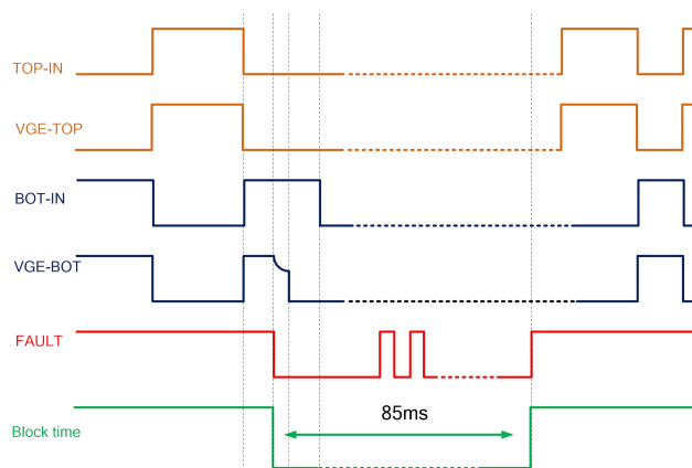
图 9 故障通信原理图
