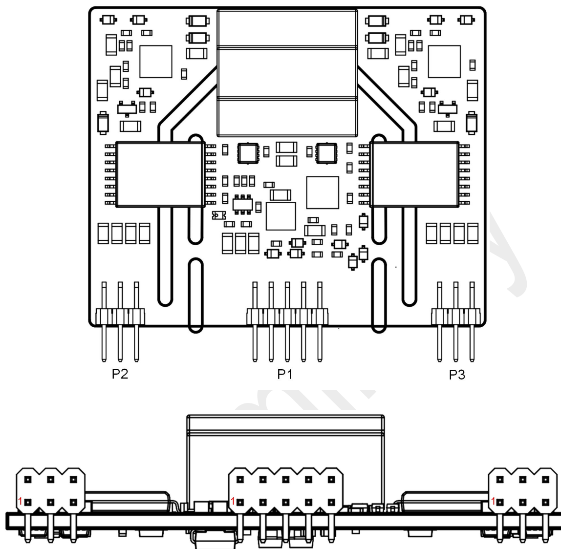
图 3 接口定义图
