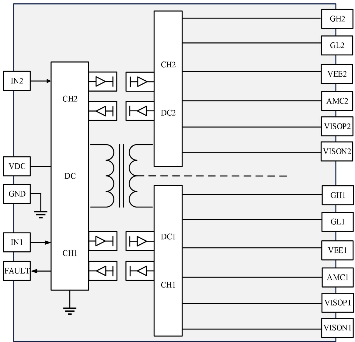
图 2 功能框架图
