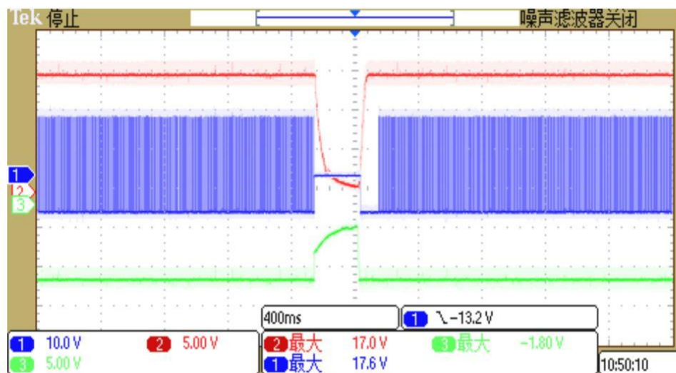
图 12 GE 短路
