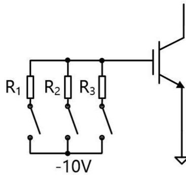
图 10 分级关断原理图
