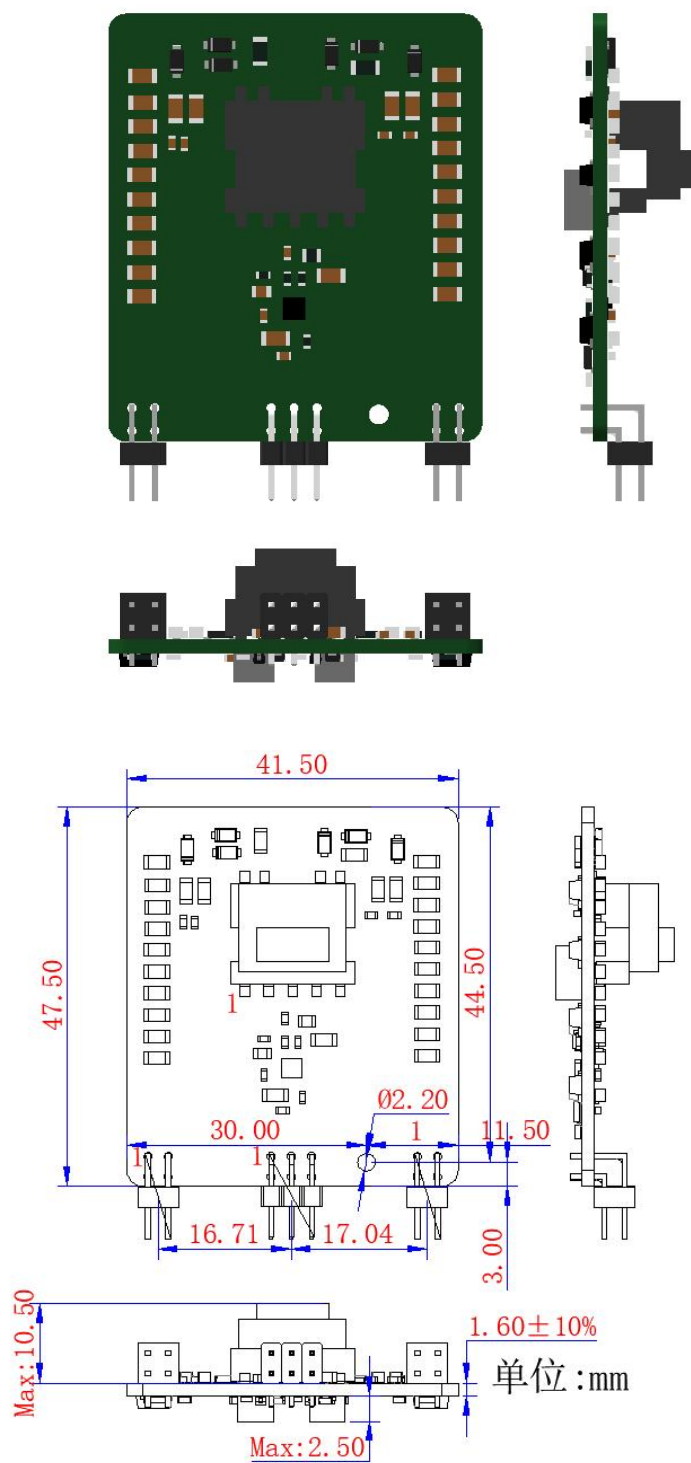
图3 3D 及机械尺寸图
