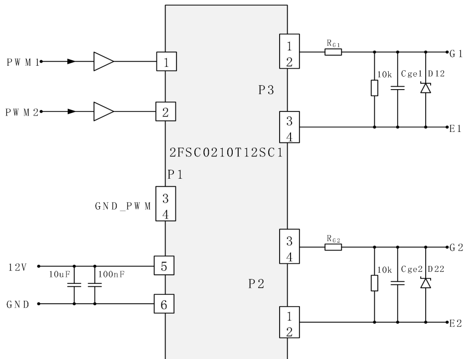
图 5 2FSC0210T12SC1 典型应用图
