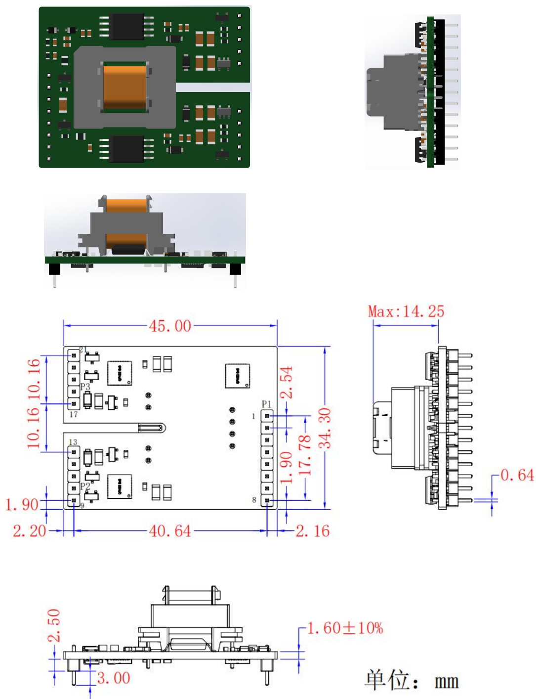
图 3 3D 和尺寸图
