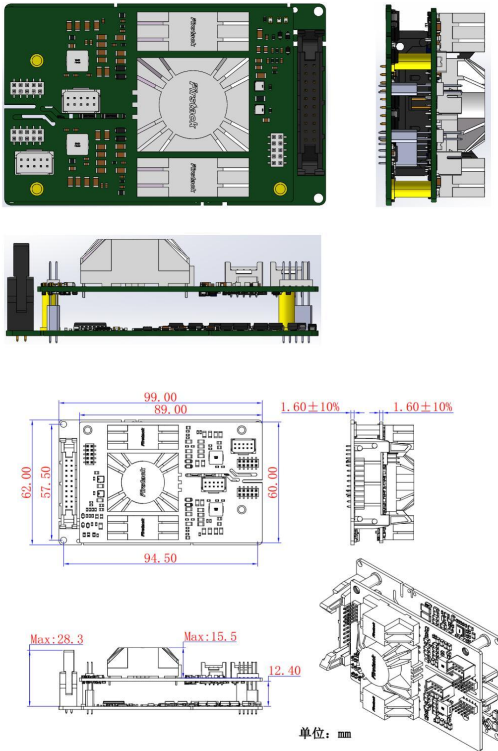
图4 3D 机械结构图
