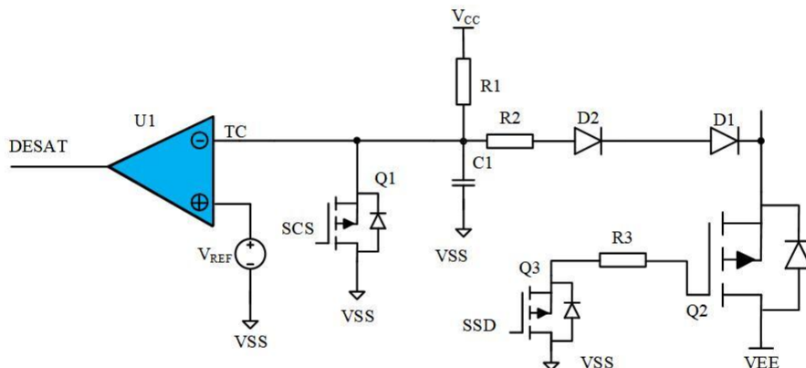
图 5 短路保护检测电路
