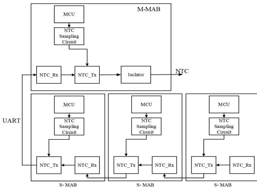
图 9 分布式 NTC 采样电路拓扑
