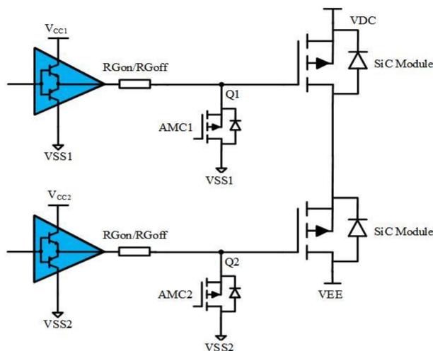
图 7 有源米勒钳位电路
