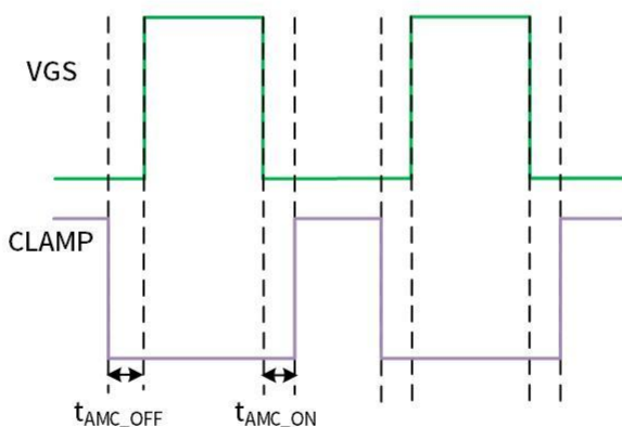
图 8 有源米勒钳位时序图
