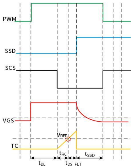
图 6 短路保护及软关时序图
