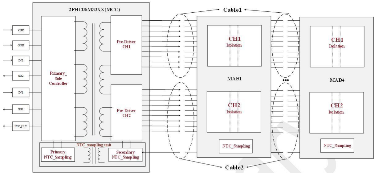
图 2 功能框架图
